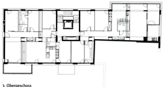
3. Obergeschoss
