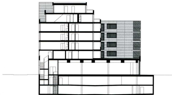
Querschnitt
