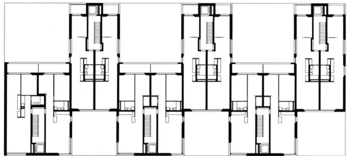
Regelgeschoss
